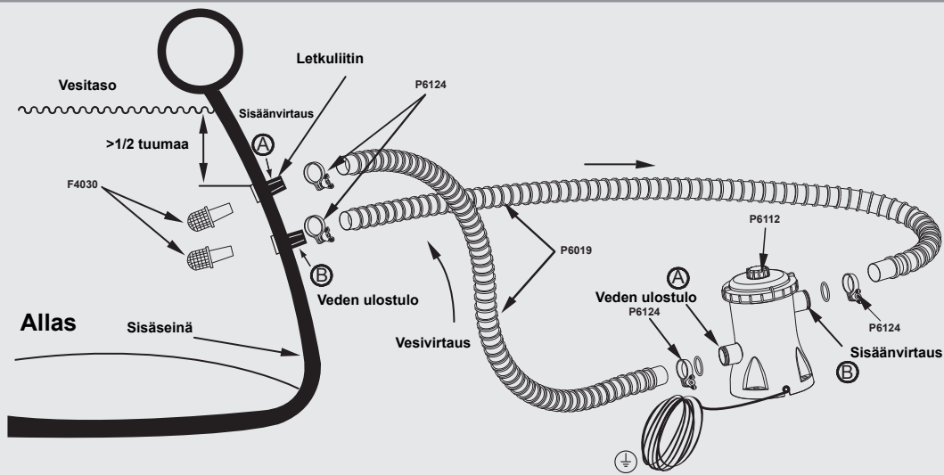
Uimaaltaan ja ROUCLAR™ suodatinpumpun kuva (ei mittakaavassa)
