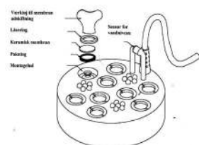
Byte av membran
